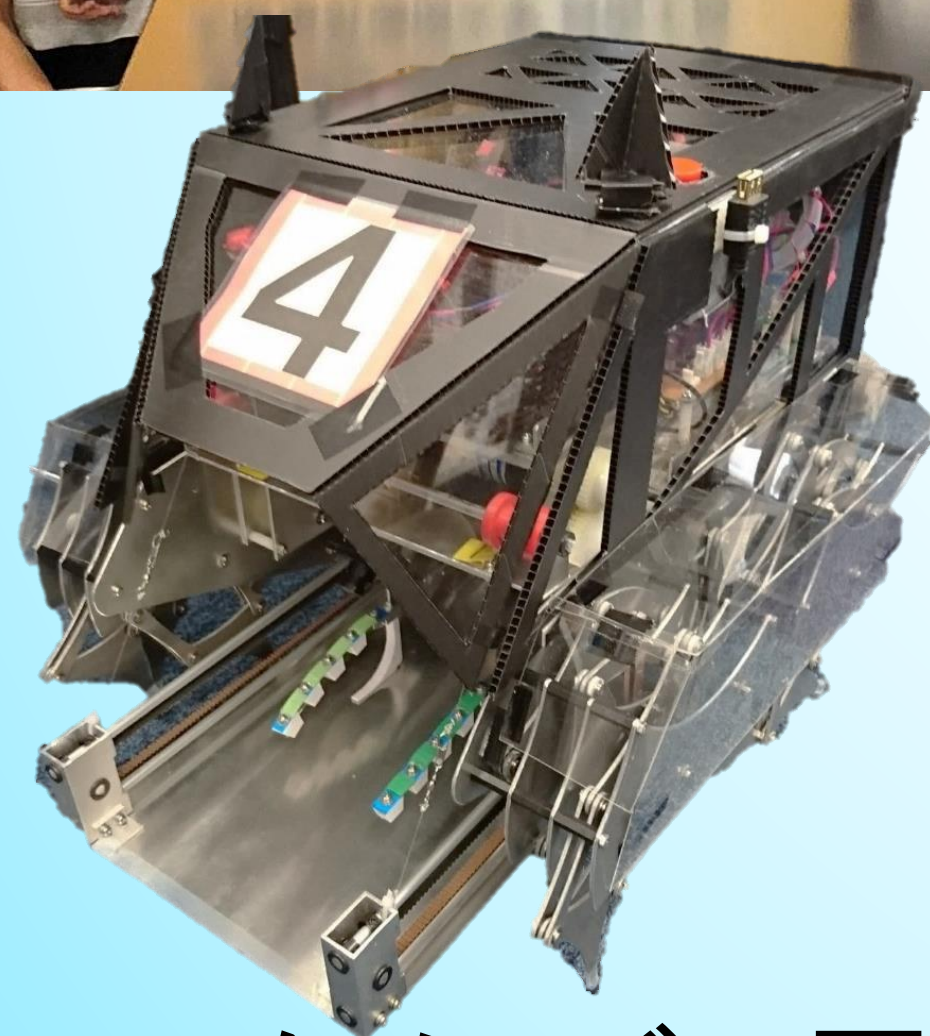
上:チームメンバー写真 下:4号機 スレイプニル
