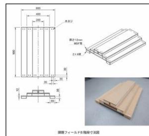
階段詳細
